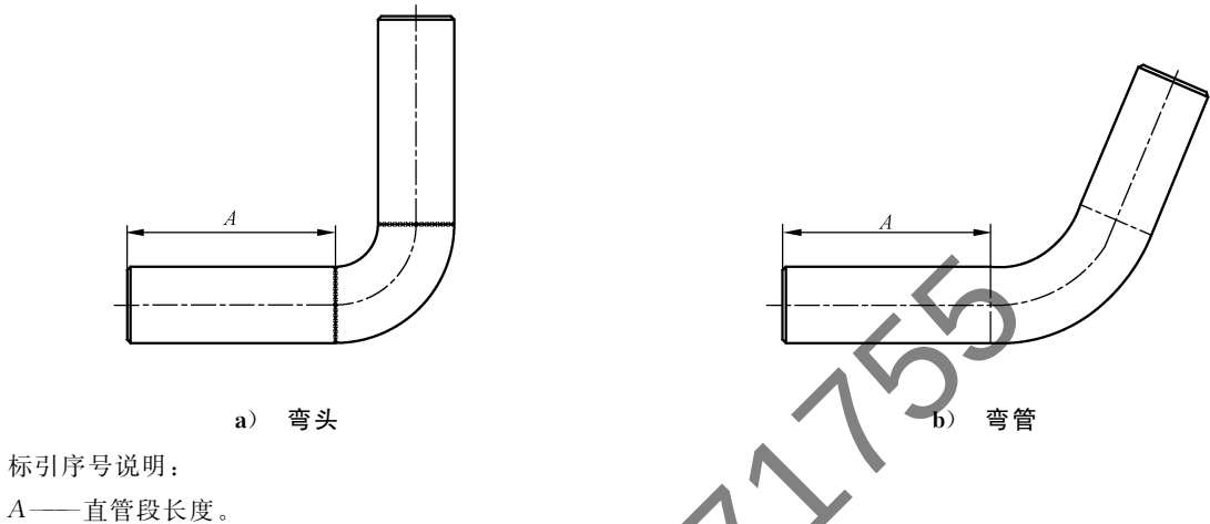
图 2 弯头与弯管管件示意
