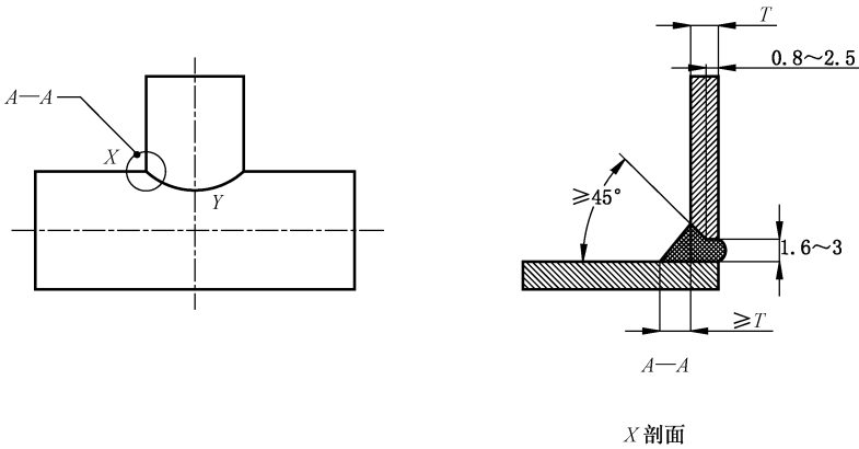
a) 不等径支管
