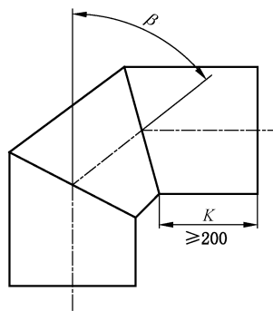
b) \beta \leq 45^\circ 三个焊接管段
