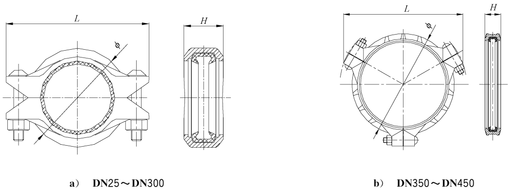
图 C.3 柔性管接头
